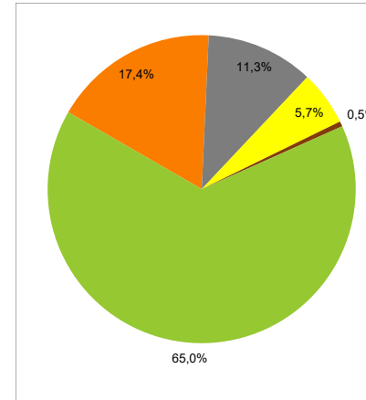
Verbleibender Energieträgermix
