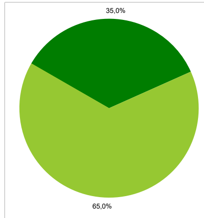
Produktmix Ökostrom
